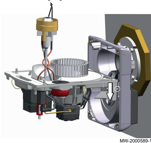
Abb.120 Reinigung des Gebläses
