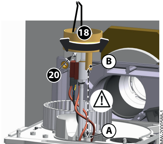
Abb.120 Reinigung des Gebläses
