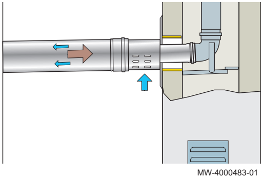
Abb.39 Anschluss vom Typ B 23P – in Frankreich innerhalb der Wohnung/des Wohnhauses anwendbar
