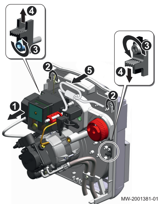
Abb.118 Austausch der Öldüse
